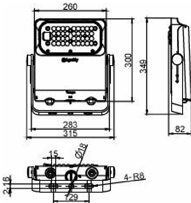
BVP561 LED163/740 100W GL SMB P7
