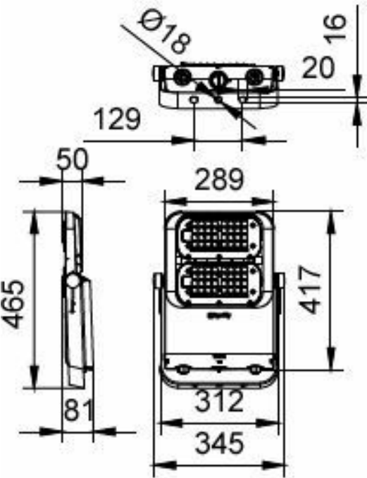
BVP562 LED270/740 155W PSU SMB
