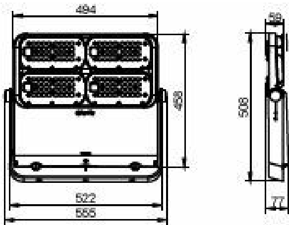
BVP562 LED270/740 155W PSU SMB
