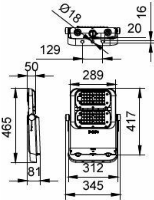
BVP562PC LED283/740 200W FP NB
